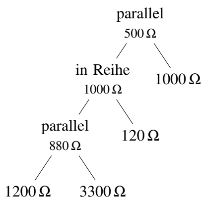
Abbildung 5.1: Darstellung des Beispiels aus der Aufgabenstellung als Baum.
